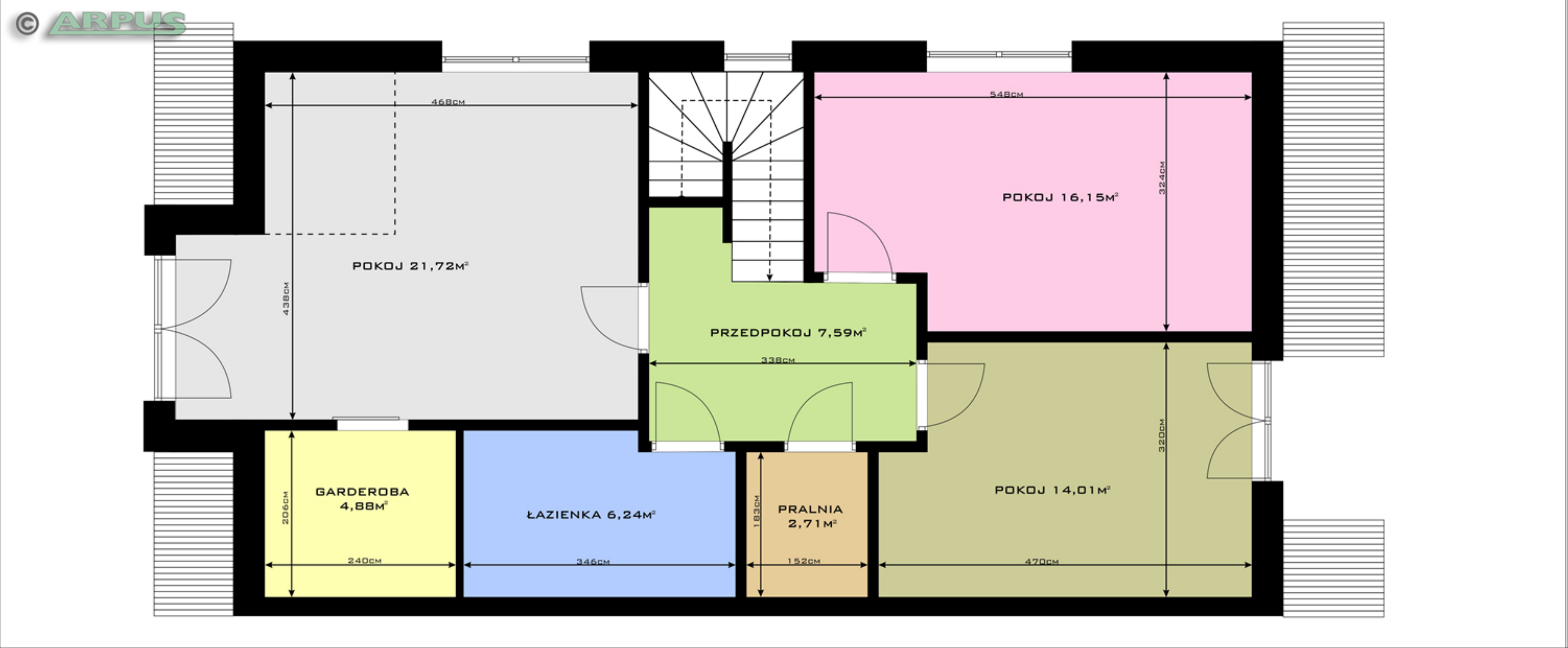
BUDYNEK B - Piętro
