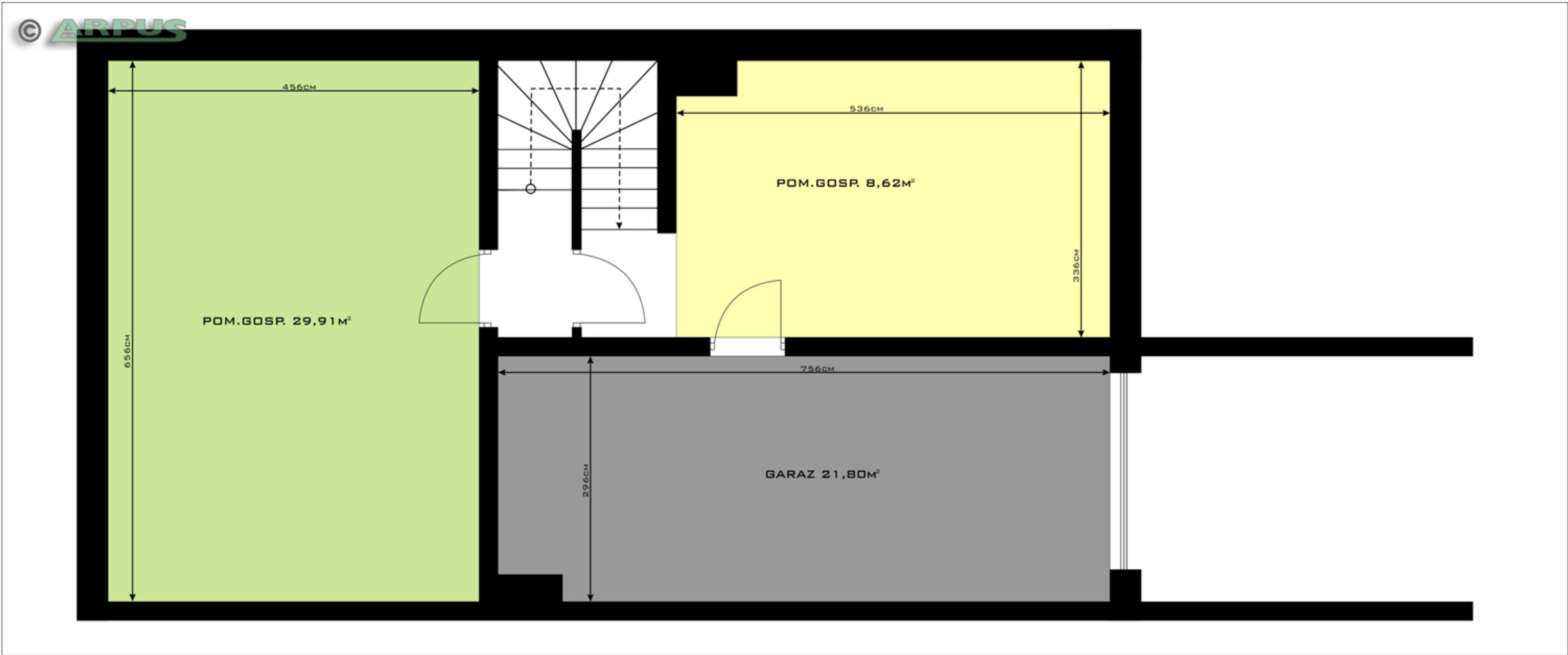
BUDYNEK B - Piwnica
